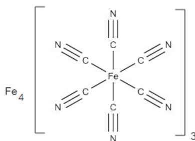
Fig. 15: Azul da prússia
