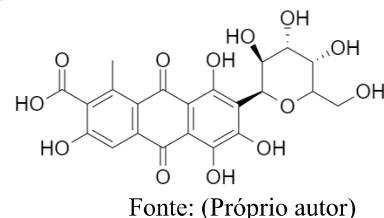
Fig. 9: Estrutura do ácido carmínico
