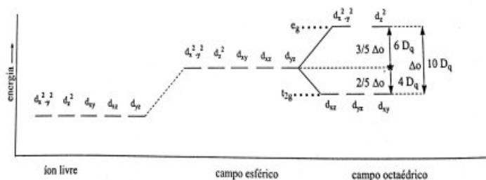
Fig. 4: Diagrama do desdobramento dos orbitais d em campo octaédrico
