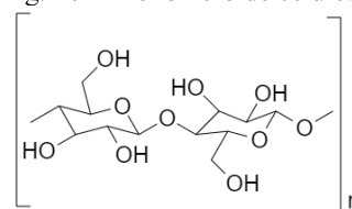
Fig. 28 – Monômero de celulose
