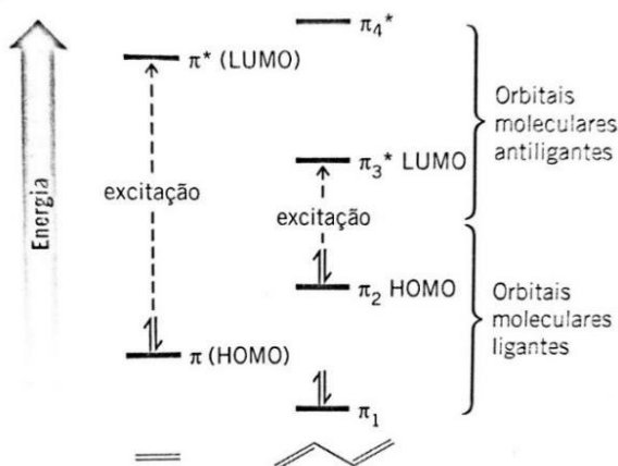
Fig. 6: Energias relativas dos orbitais \pi do eteno e do 1,3-butadieno
