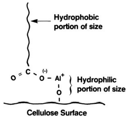
Fig. 29: Interação do agente coagulante com a fibra de celulose e a colofônia
