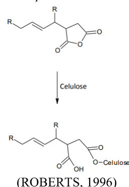
Fig. 31: Reação entre celulose e AKD
