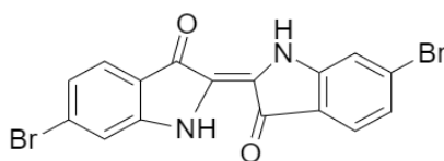
Fig.8: Estrutura do corante “púrpura tíria”
