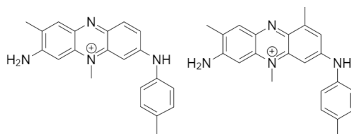
Fig. 19: Moléculas presentes no pigmento “malve”
