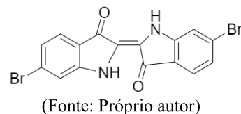
Fig.8: Estrutura do corante “púrpura tíria”
