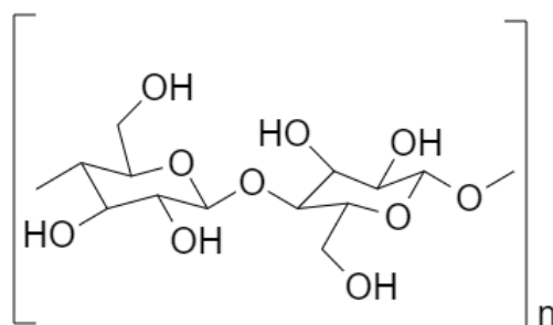
Fig. 28 – Monômero de celulose
