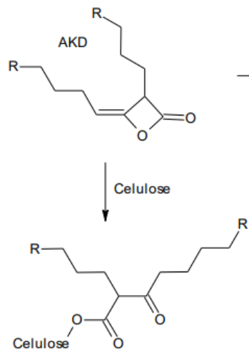
Fig. 31: Reação entre celulose e AKD
