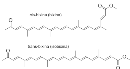
Fig. 10: Moléculas de bixina e isobixina
