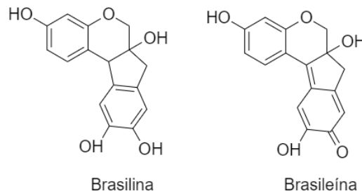
Fig. 11: Moléculas brasileína e brasilina
