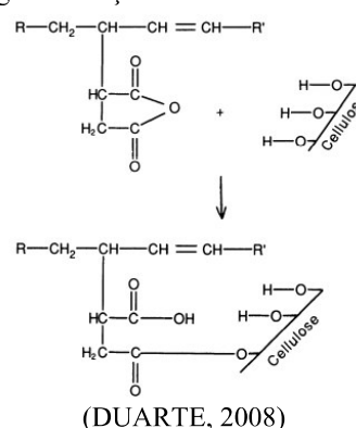
Fig. 32: Reação entre celulose e ASA
