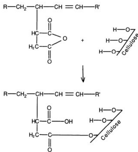
Fig. 32: Reação entre celulose e ASA
