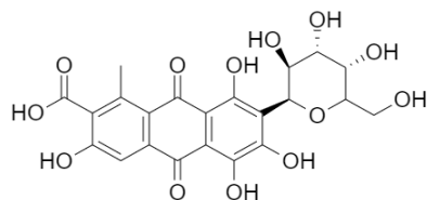
Fig. 9: Estrutura do ácido carmínico
