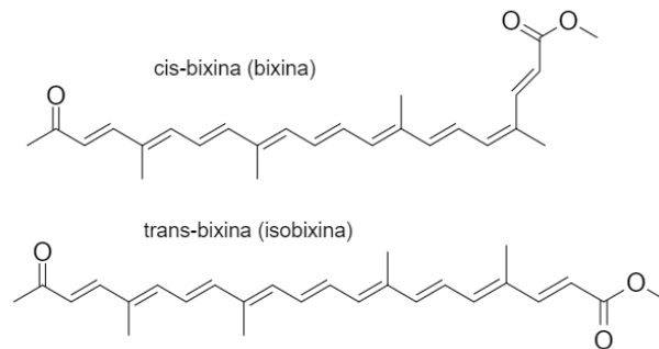
Fig. 10: Moléculas de bixina e isobixina
