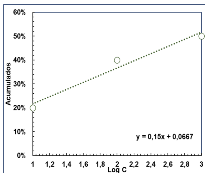
Figura 1: Percentual de mortalidade de Artemia salina versus o log da concentração do OE
