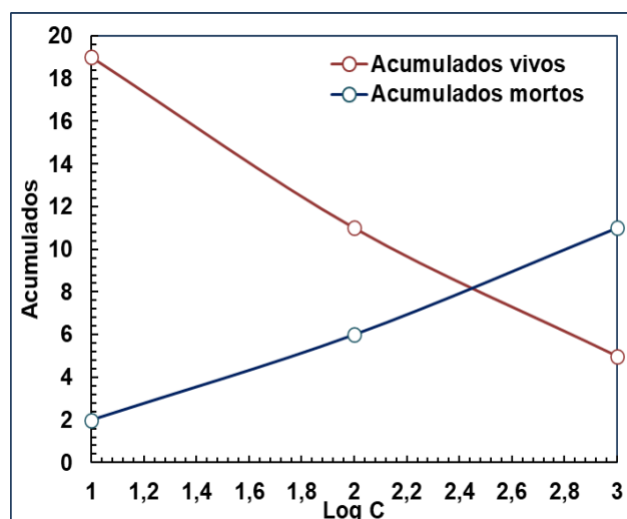
Figura 2: Gráfico log da concentração do OE versus os acumulados de Artemia salina
