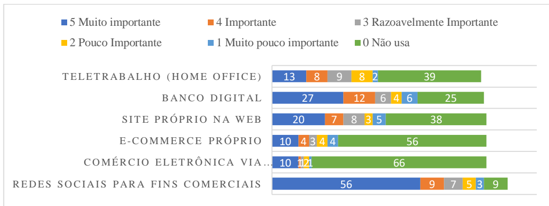
Gráfico 3 - Avaliação do grau de importância das tecnologias básicas citadas na pesquisa
